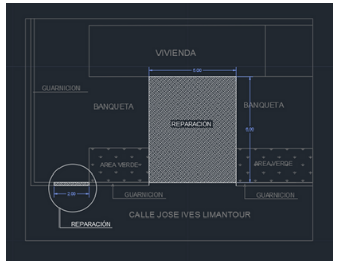
(Planta en AutoCAD para reparación de banqueta y/o guarnición)
