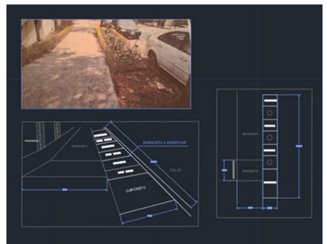
(Planta en AutoCAD para reparación de banqueta y/o guarnición)
